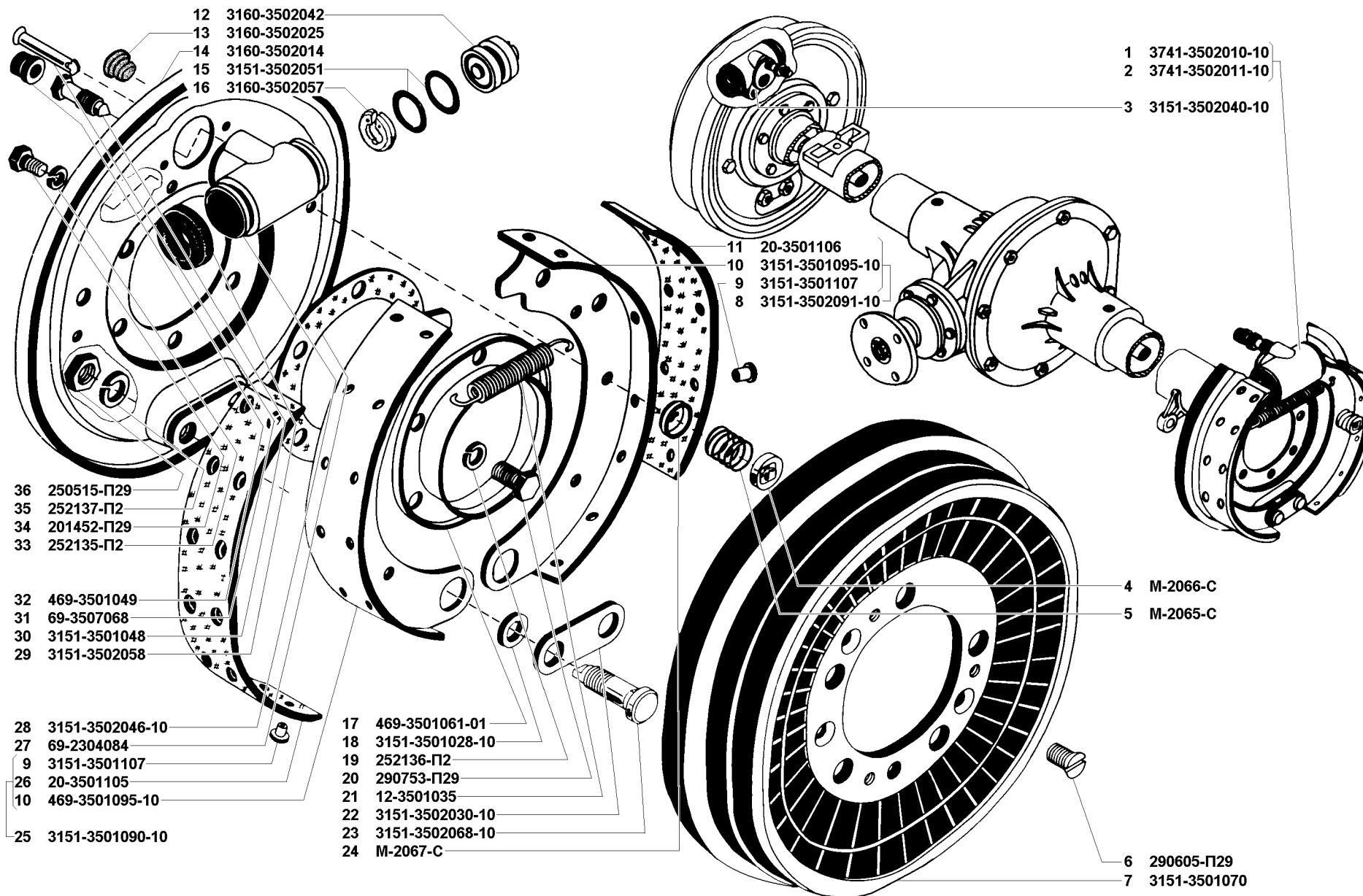
Рис. 81. Тормоза рабочие задние и тормозные барабаны (3502)+
